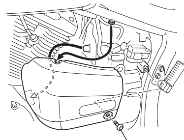
取付ボルト
