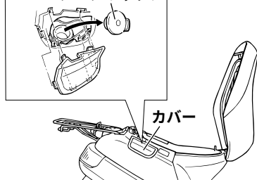
オイルタンクキャップ
