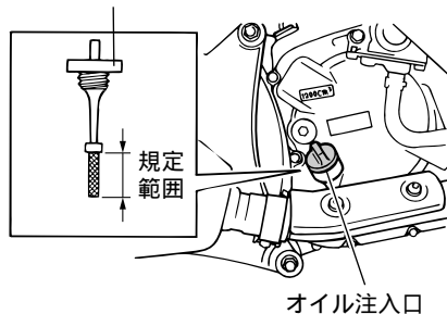
オイルレベルゲージ
