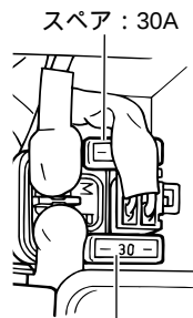
メインヒューズ : 30A
