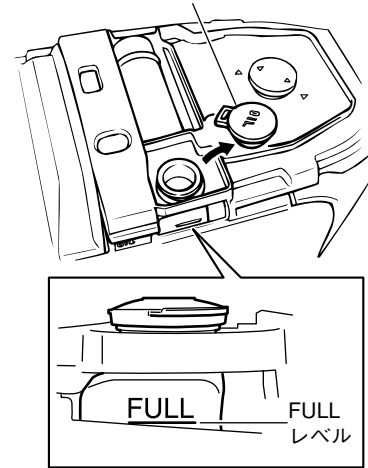
オイルタンクキャップ
