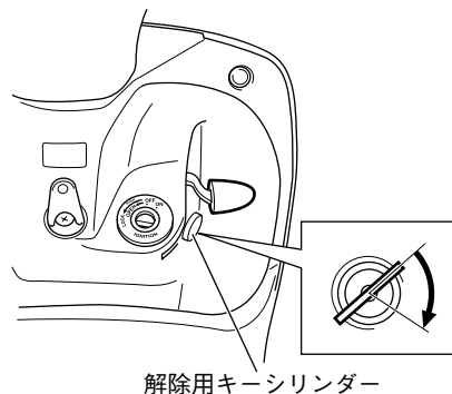
解除用キーシリンダー
