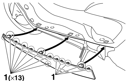
1. ツメ
