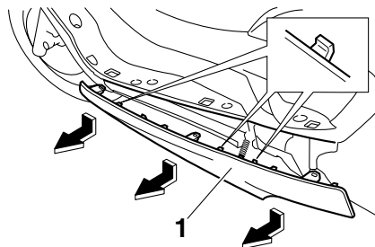
1. カバー A
