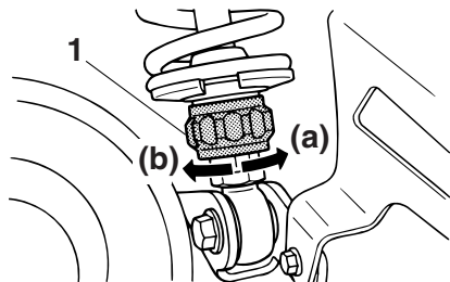
1. 伸側減衰力アジャスター
