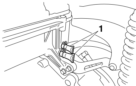
1. ブローバイガス選元装置のブリーザー dren ホース
