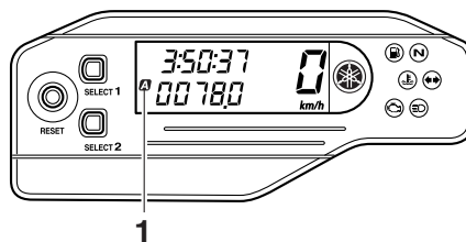
1. トリップメーター A 表示 “A”
