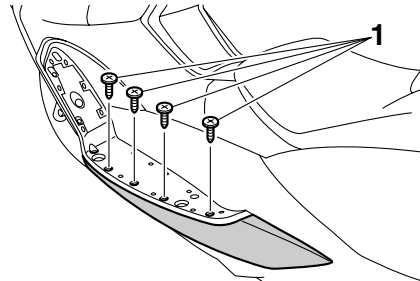
1. スクリュー
