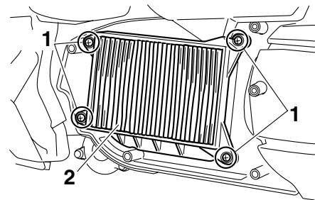
1. スクリュー 2. V ベルトフィルターエレメント
