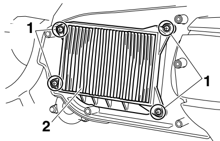
1. スクリュー
