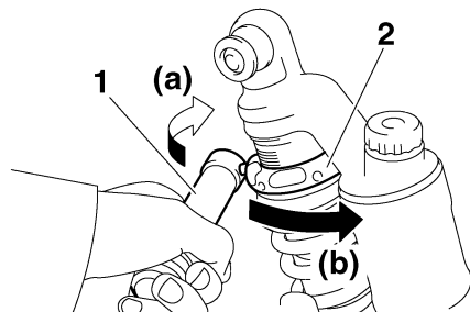
1. 調整レンチ 2. スプリングプリロードアジャスター
