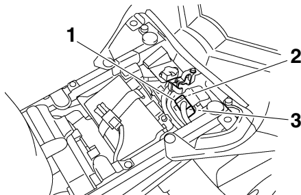
1. スターターリレーカバー 2. フューエルインジェクションヒューズ 3. スペアフューエルインジェクションヒューズ
