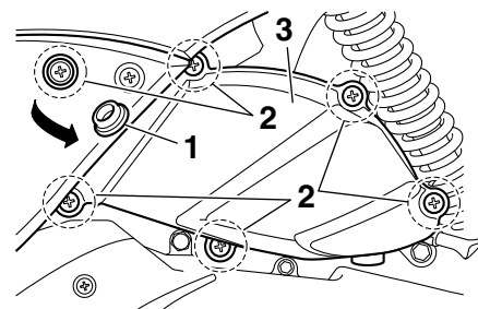
1. カバー 2. スクリュー 3. エアクリーナーケースカバー
