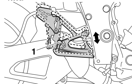
1. フットレスト
