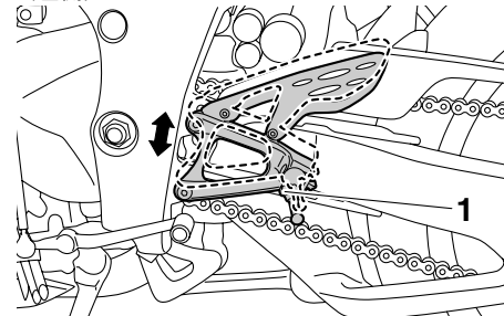
1. フットレスト
