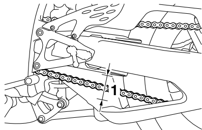
1. ドライブチェーンのたわみ量
