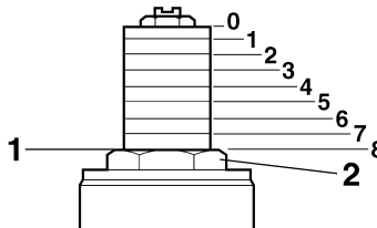
1. 調整位置 2. フロントフォークキャップボルト
