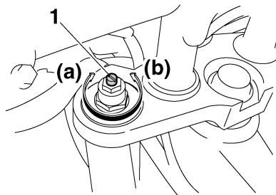
1. 圧側減衰力アジャスター
