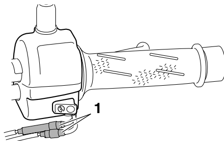
1. ゴムカバー
