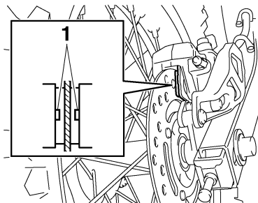
1. インジケータ溝
