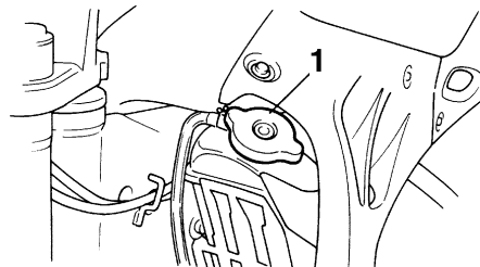
1. ラジエーターキャップ
