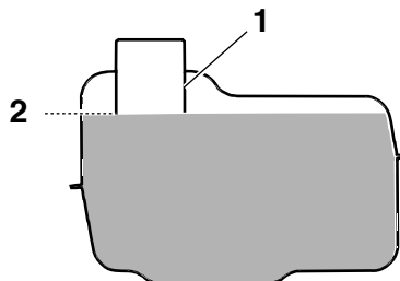
1. フィラーチューブ 2. 給油限度
