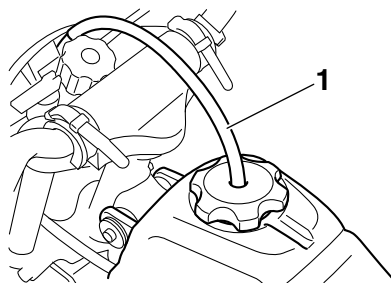
1. フューエルタンクブリーザーホース
