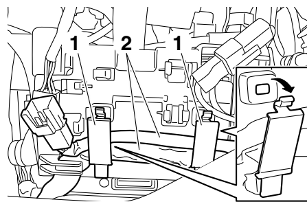
1. クランプ 2. ワイヤーハーネス
