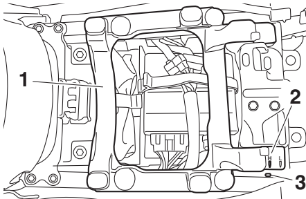
1. ライダーシートハイトアジャスター 2. “H” マーク 3. 合マーク
