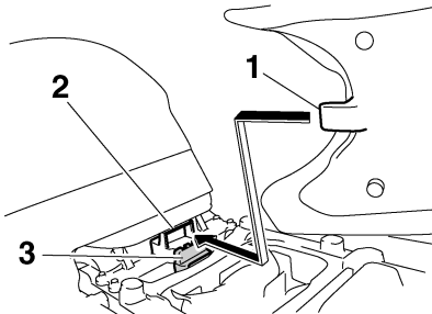
1. 突起 2. シートホルダー B (高い位置用) 3. ライダーシートホルダーカバー
