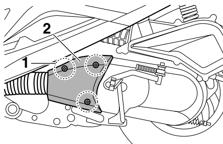
1. スクリュー 2. V ベルトフィルターケースカバー
