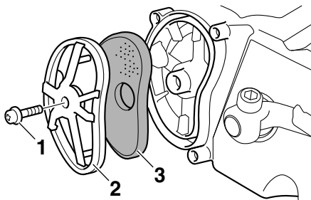
1. スクリュー 2. V ベルトフィルターエレメントホルダー 3. V ベルトフィルターエレメント
