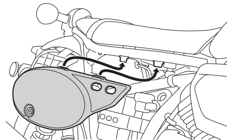
カバ－C
