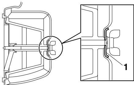
1. ワッシャー
