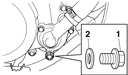
1. 冷却水ドレンボルト
