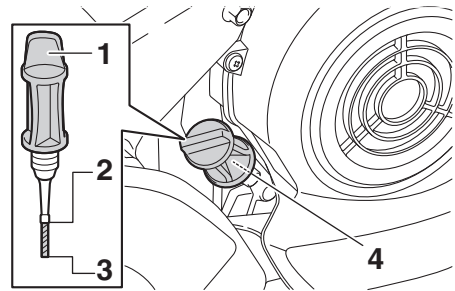
1. オイルレベルゲージ 2. フルレベル 3. ロアレベル 4. オイル注入口
