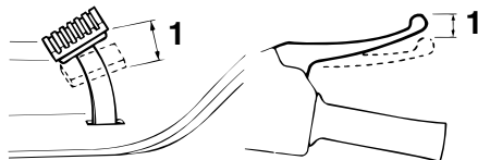
<リアブレーキ>
