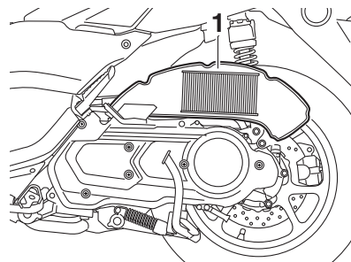
1. エアクリーナーエレメント
