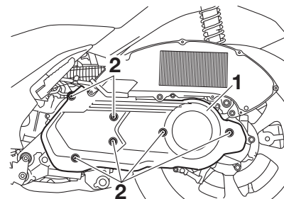
1. Vベルトフィルターケースカバー 2. スクリュー
