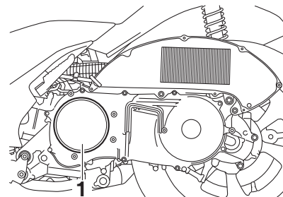
1. Vベルトフィルターエレメント
