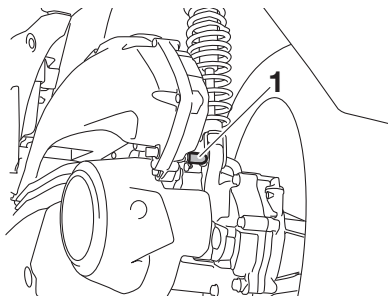
1. ブローバイガス還元装置のブリーザー drenホース
