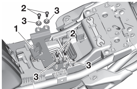
1. シートホルダー 2. ボルト 3. ワッシャー
