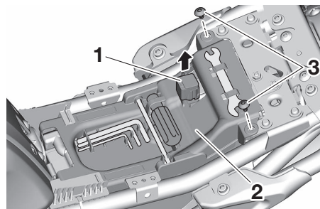
1. 故障診断コネクタ 2. バッテリーカバー 3. ボルト
