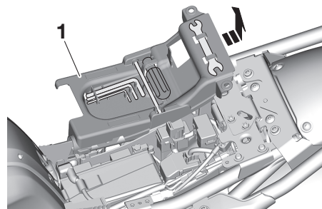
1. バッテリーカバー
