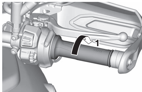
1. 減速方向
