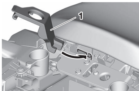
1. キャップ
