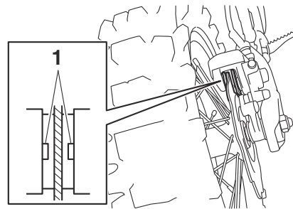
1. インジケータ溝
