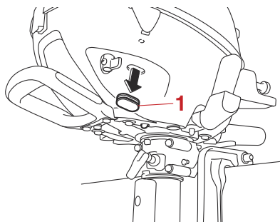
1. グロメット
