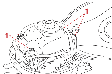
1. ボルト
