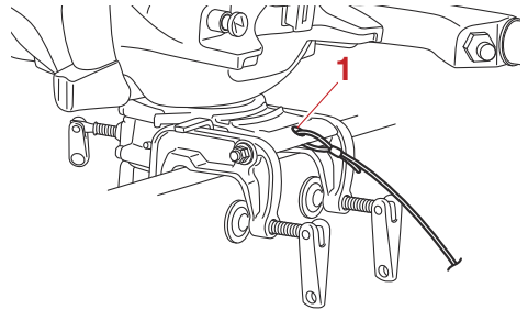
1. 係船ロープアタッチメント
