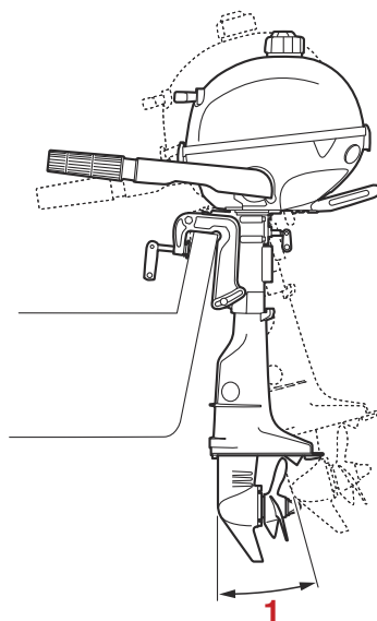
1. トリム範囲
