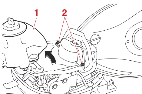
1. 燃料タンク 2. ボルト
