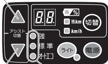
走行モード切替ボタン“▽” (アシストダウン)
